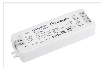
Блок управления «неоном» от пульта и панели
