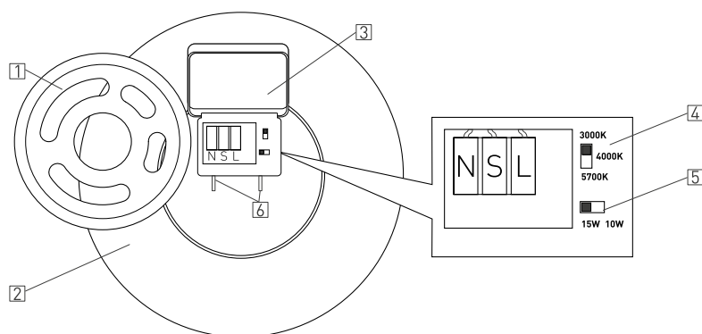
Рис. 2. Установка и настройка светильника
