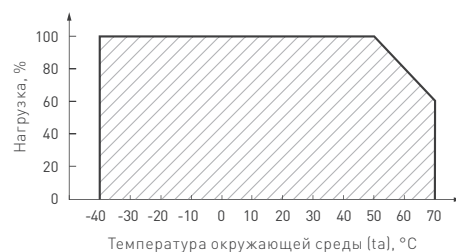
Рис. 2. Максимальная допустимая нагрузка, % от мощности источника
