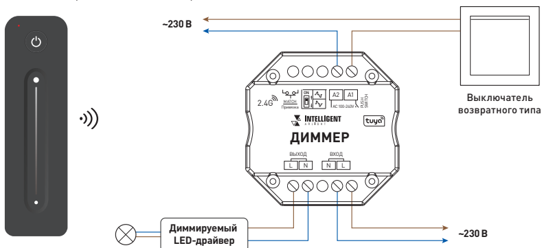
Рис. 1. Схема соединения оборудования
