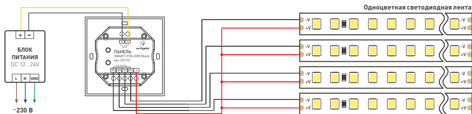
Рис. 1. Подключение одноцветной светодиодной ленты
