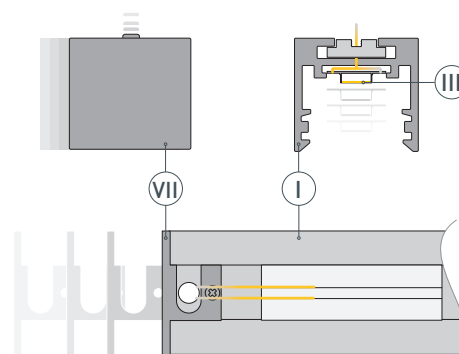
Рис. 1. Установка заглушки ⑦ на профиль ①. Вид сверху
