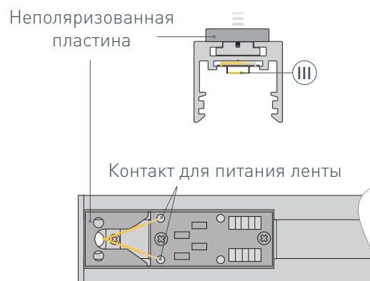
Рис. 2. Неполяризованная пластина на профиле ①. Вид сверху
