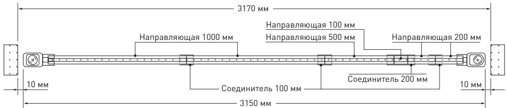
Рис. 4. Пример сборки направляющей длиной 3.15 м
