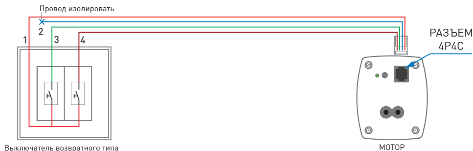
Рис. 7. Подключение мотора с помощью «сухих контактов»
