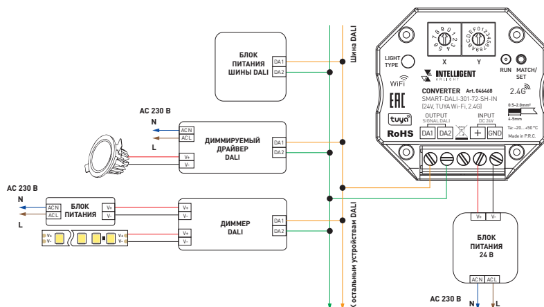
Рис. 1. Схемы подключения диммера
