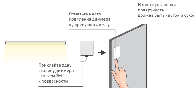
Рис. 2. Установка диммера SR-PRIME-UP
