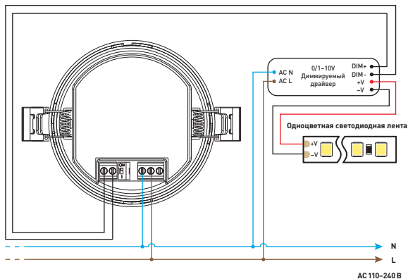
Рис. 2. Схема подключения датчика движения к диммеру с управлением 0/1-10 В
