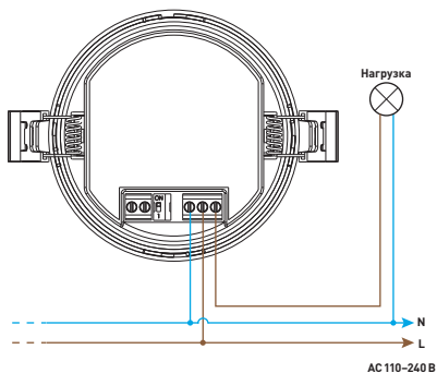
Рис. 1. Схема подключения датчика движения к не диммируемому источнику света (AC 100-240 В)
