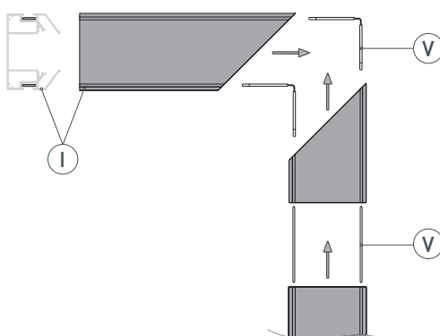
Рис. 1. Виды соединений
